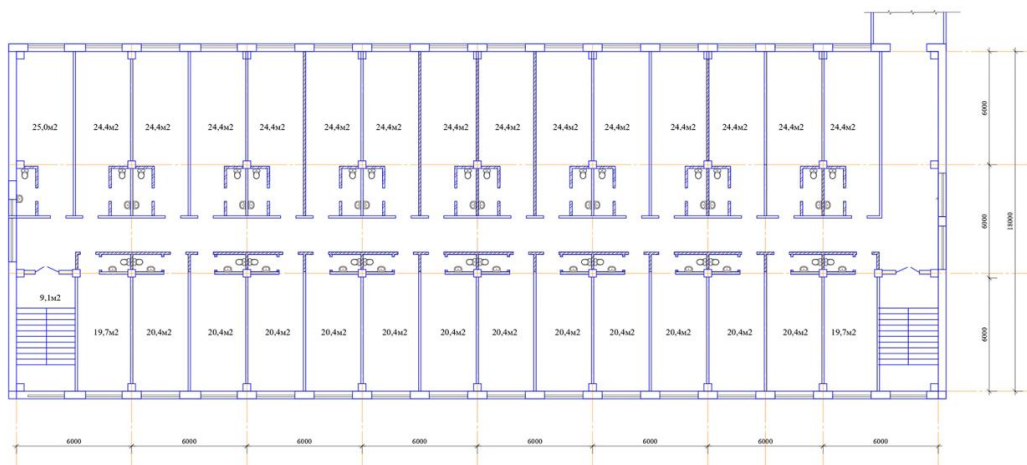
ПОВЕРХОВИЙ ПЛАН БУДІВЛІ ОФІСНОГО ЦЕНТРУ ISATEX
